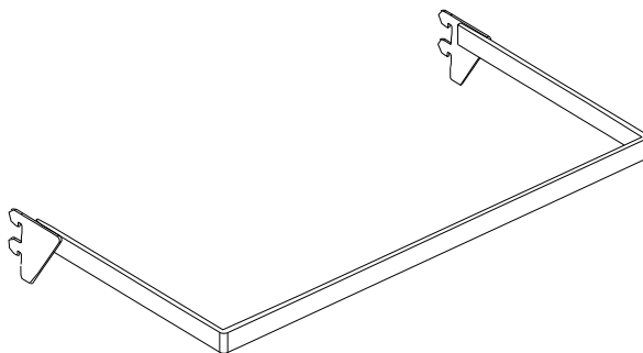
Hak konfekcyjny z płaskownika, tzw. obręcz szer: 600mm gł: 300mm
